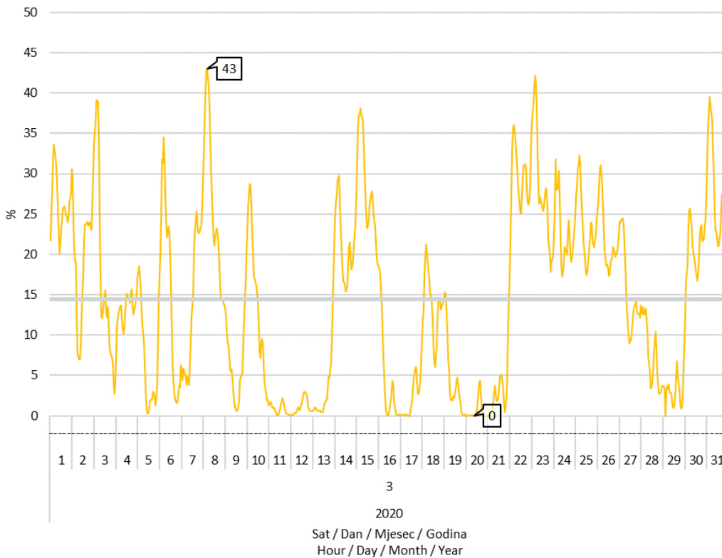
Slika 8 Udio proizvodnje vjetroelektrana u pokrivanju satnog opterećenja elektroenergetskog sustava u ožujku 2020. godine
