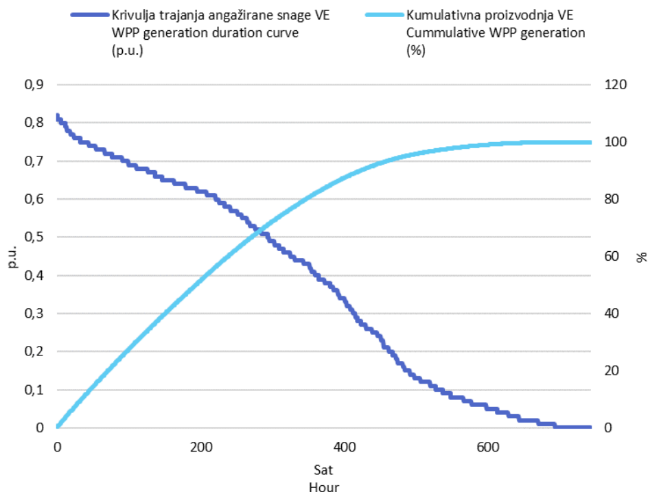
Slika 3 Krivulja trajanja angažirane snage svih VE i kumulativna proizvodnja VE u ožujku 2020. godine u jediničnim vrijednostima
