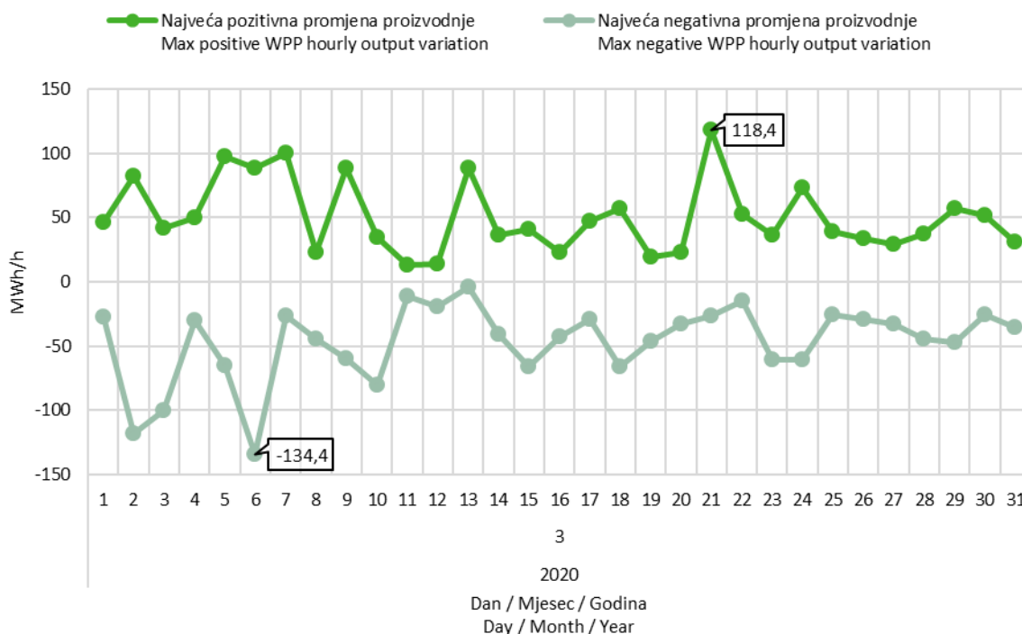
Slika 9 Maksimalna pozitivna i maksimalna negativna promjena satne proizvodnje VE u ožujku 2020. godine
