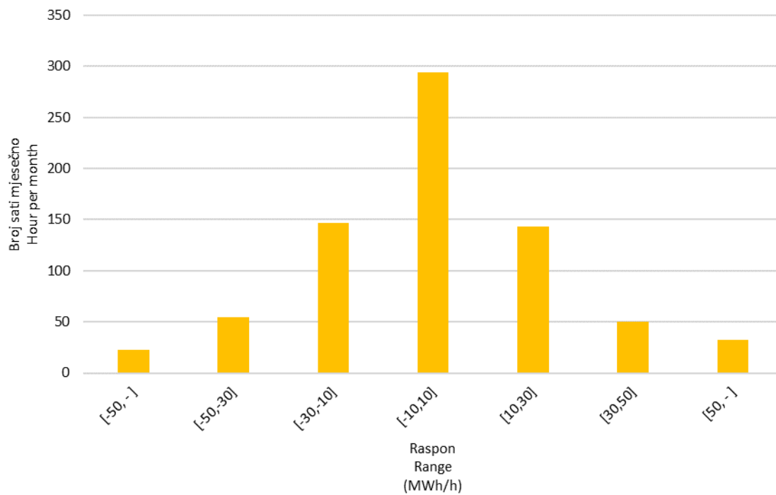
Slika 10 Statistička raspodjela satnih promjena proizvodnje VE u ožujku 2020. godine Figure 10 Statistical distribution of WPP hourly output variations in March 2020
