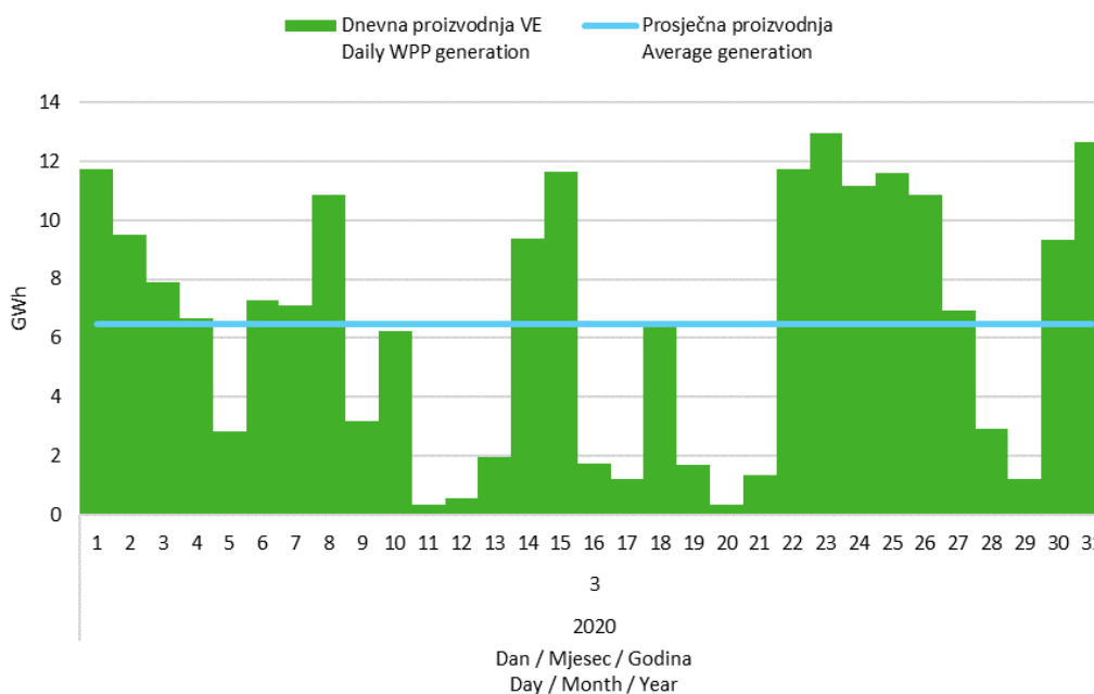
Slika 5 Dnevna proizvodnja svih vjetroelektrana u ožujku 2020. godine
