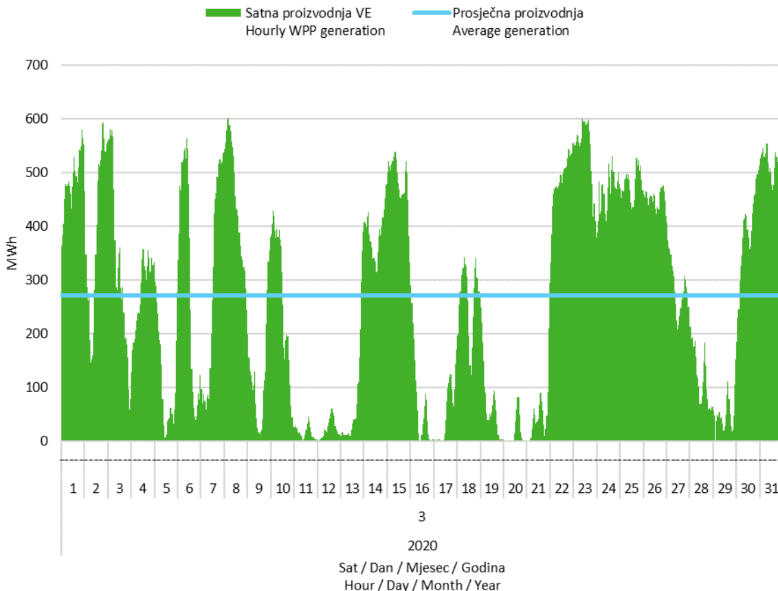
Slika 2 Satna proizvodnja svih vjetroelektrana u ožujku 2020. godine
