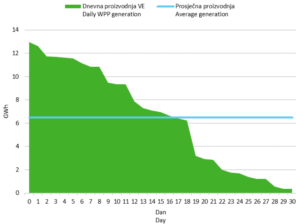
Slika 6 Krivulja trajanja dnevne proizvodnje vjetroelektrana u ožujku 2020. godine
