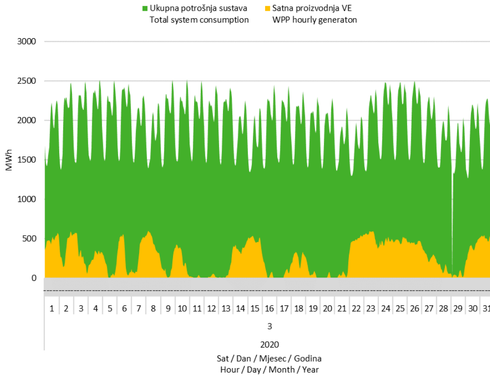
Slika 7 Usporedba satnog dijagrama opterećenja sustava i proizvodnje vjetroelektrana u ožujku 2020. godine
